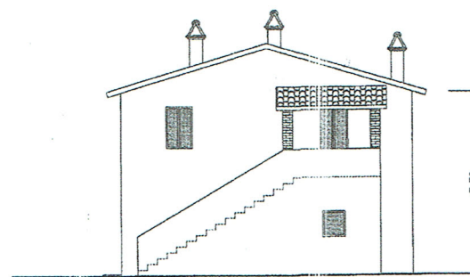
PROSPETTO NORD
