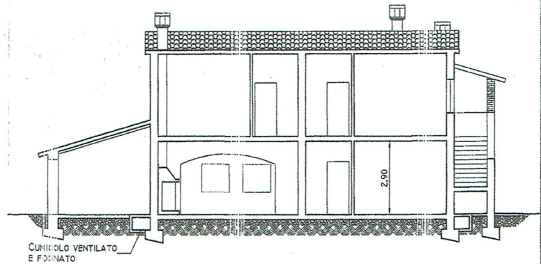
SEZIONE B-B'
