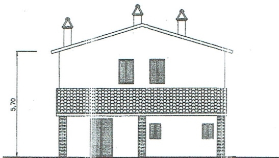
PROSPETTO SUD
