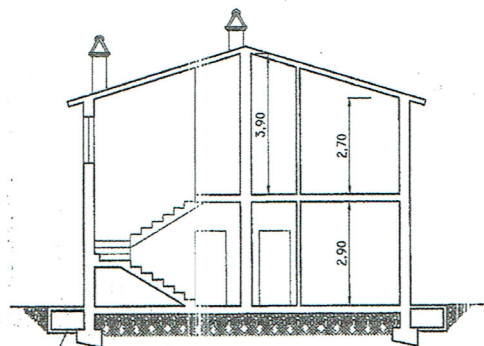
SEZIONE A-A'
