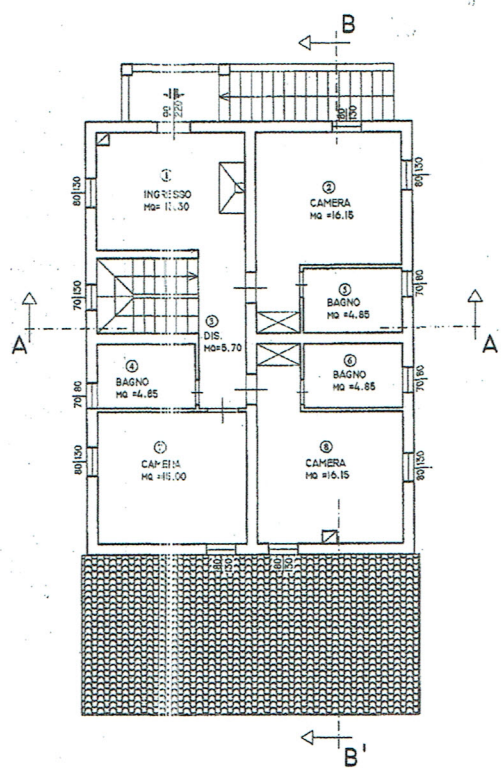
PIANO PRIMO
