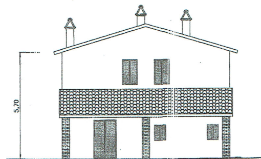
PROSPETTO SUD
